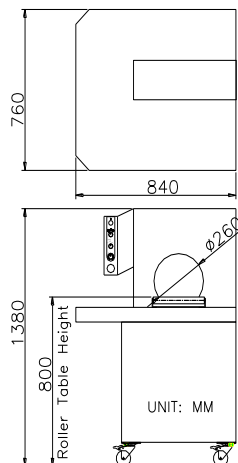
機械外型圖
