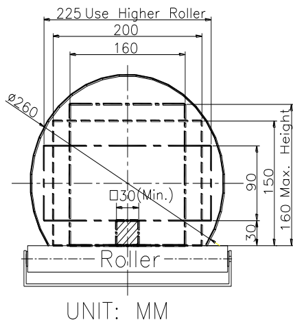
裹包範圍圖
